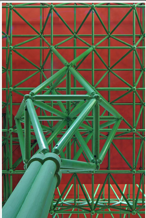
Stahlrohr-Tragewerk (MERO)
